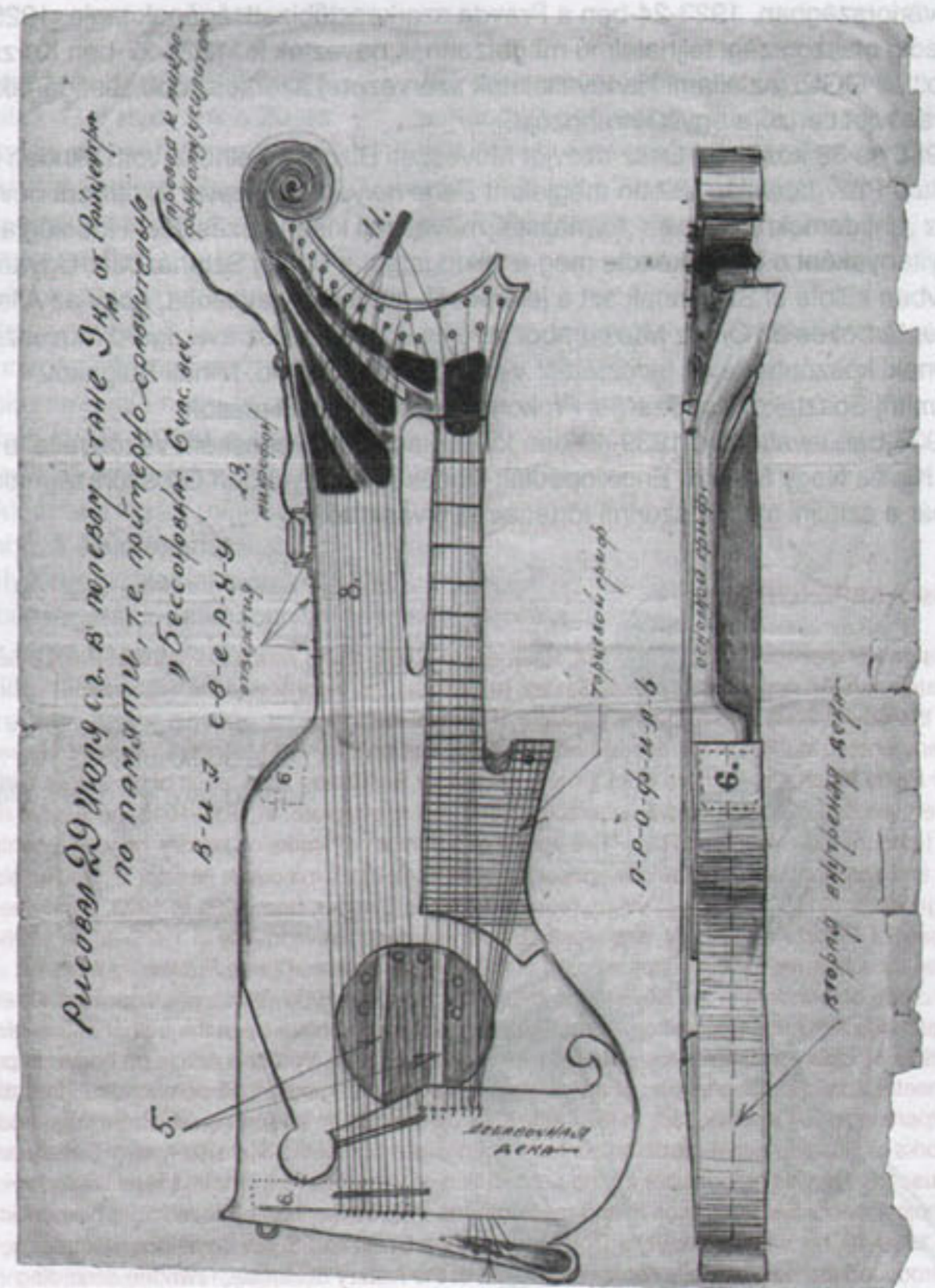
A 23 húrú elektromos gitár tervrajza, 1935. augusztus 6., a Theremin Központ archívuma Plan for construction of a 23-string electrified guitar. August 6, 1935. Theremin Center archive
